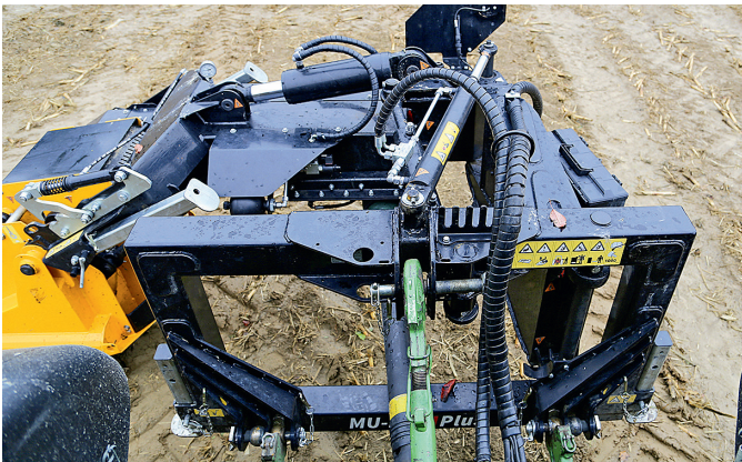
Masyvus pakabinimo rėmas gerai matomas iš operatoriaus darbo vietos. Kaip ir kituose Müthing smulkintuvuose, taip ir MU-M/S Plus Vario 220 naudojamas stačiakampio formos rėmas iš uždarytą kvadratinio profilio vamzdžių
